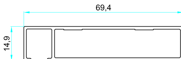
Premarco 70 mm 8265 Peso: 0,552 kg/m
