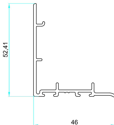
Cruce de hojas 8219 Peso: 0,496 kg/m
