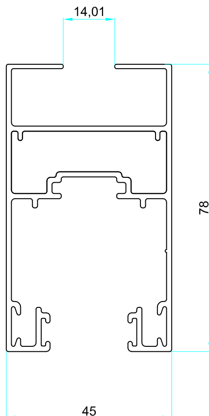
Hoja corte a 45° V.Simple 8251 Peso: 1,342 kg/m
