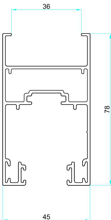
Hoja corte a 45° DVH 8222 Peso: 1,270 kg/m
