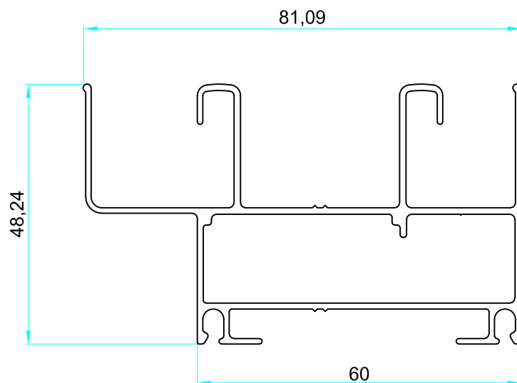
Marco 60 mm corrediza c caja de agua 8056 Peso: 1,030 kg/m
