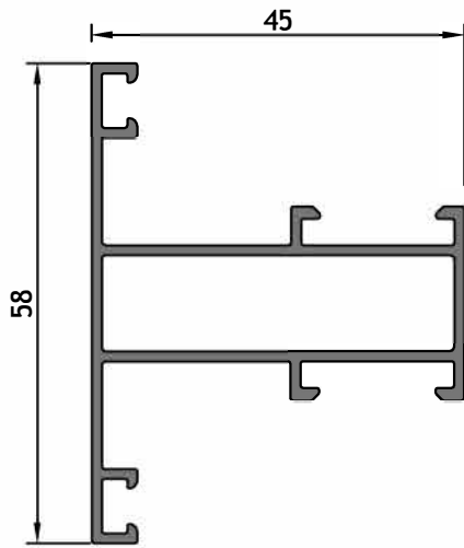
AM - 221 Travesaño angosto pañó fijo Peso: 0,767 kg/m Largo: 6150 mm Paquete x 4 tiras
