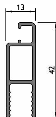
AM-255 Bastidor de mosquitero Peso: 0,389 kg/m Largo: 6150 mm Paquete x 10 tiras
