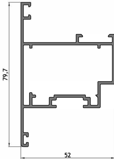
AM - 258 Hoja ventana proyectante recta Peso: 1,061 kg/m Largo: 6150 mm Paquete x 2 tiras
