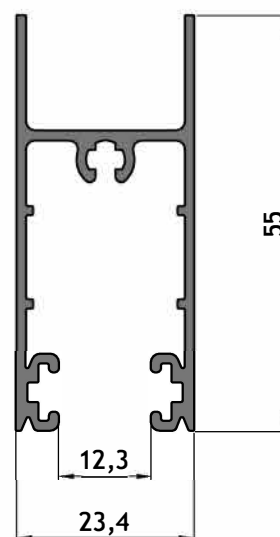
AM - 249 Cabezal / zócalo DVH Peso: 0,632 kg/m Largo: 6150 mm Paquete x 6 tiras
