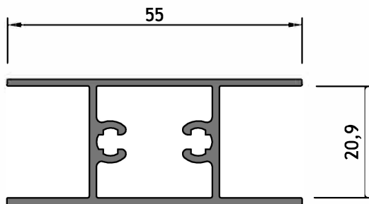
AM - 253 Travesaño de puerta corrediza para DVH
