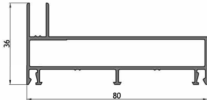
AM - 241 Jamba marco 80 Peso: 0,969 kg/m Largo: 6150 mm Paquete x 2 tiras
