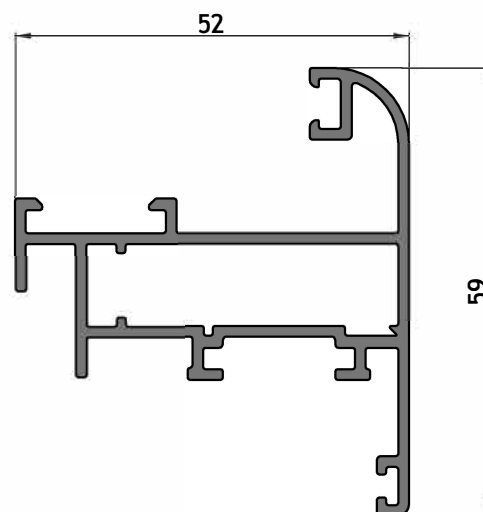
AM - 236 Hoja curva ventiluz curva Peso: 0,902 kg/m Largo: 6150 mm Paquete x 2 tiras
