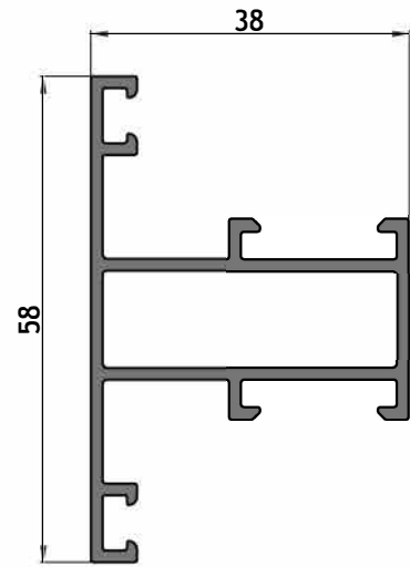
AM - 264 Travesaño para paño fijo curvo Peso: 0,713 kg/m Largo: 6150 mm Paquete x 4 tiras
