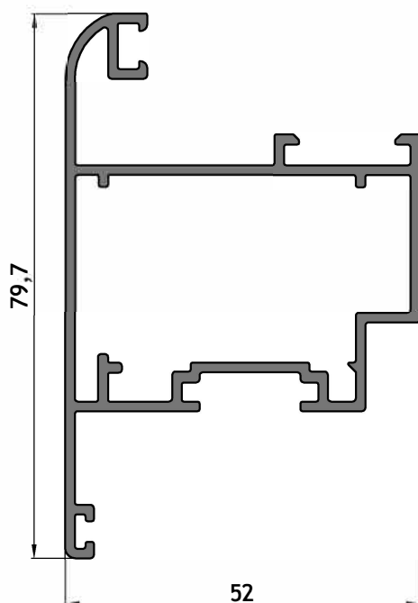
AM - 260 Hoja ventana proyectante curva Peso: 1,099 kg/m Largo: 6150 mm Paquete x 2 tiras
