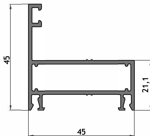
AM - 259 Marco de ventana proyectante Peso: 0,748 kg/m Largo: 6150 mm Paquete x 4 tiras
