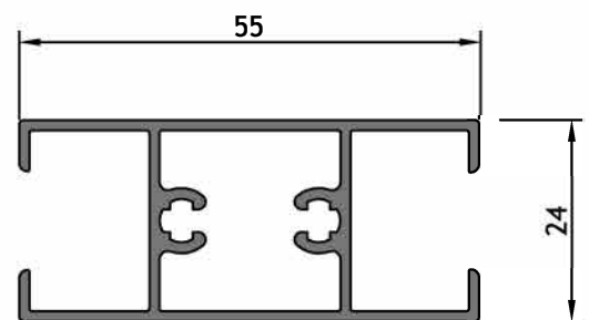
AM - 239 Travesaño hoja vidrio simple puerta corrediza
