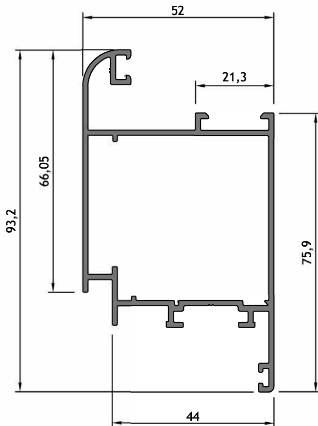
AM - 614 Hoja de puerta de 45 mm Peso: 1,194 kg/m Largo: 6150 mm Paquete x 2 tiras
