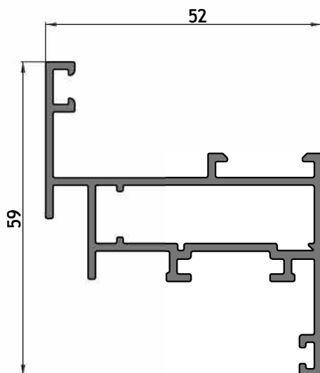
AM - 215 Hoja recta ventana de abrir doble contacto / banderola Peso: 0,861 kg/m Largo: 6150 mm Paquete x 2 tiras
