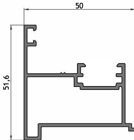
AM - 224 Encuentro central de ventana de abrir 2 hojas Peso: 0,780 kg/m Largo: 6150 mm Paquete x 2 tiras
