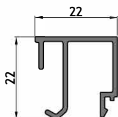
AM - 225 Contravidrio recto 22 mm Peso: 0,310 kg/ml Largo: 6150 mm Paquete x 10 tiras
