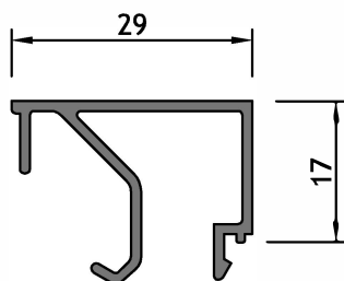
AM - 217 Contravidrio recto 29 mm Peso: 0,292 kg/m Largo: 6150 mm Paquete x 10 tiras
