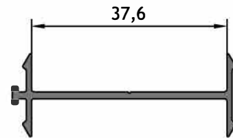
AM - 213 Acople marco Peso: 0,257 kg/m Largo: 6150 mm Paquete x 10 tiras
