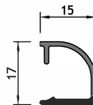
AM - 231 Contravidrio curvo DVH Peso: 0,159 kg/m Largo: 6150 mm Paquete x 10 tiras
