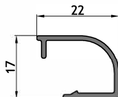
AM - 232 Contravidrio curvo 22 mm Peso: 0,181 kg/m Largo: 6150 mm Paquete x 10 tiras
