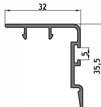
AM - 907 Complemento parante central 45° Peso: 0,381 kg/m Largo: 6150 mm Paquete x 10 tiras
