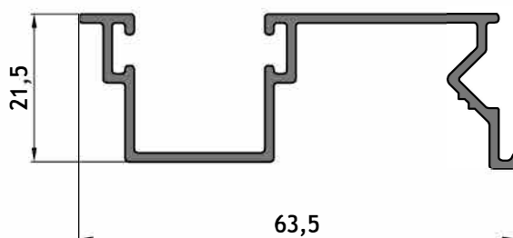
AM - 243 Guía cortina Peso: 0,545 kg/m Largo: 6150 mm Paquete x 4 tiras
