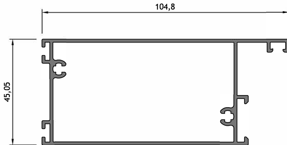
AM - 616 Zócalo de puerta de 45 mm Peso: 1,199 kg/m Largo: 6150 mm Paquete x 2 tiras
