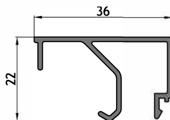
AM - 212 Contravidrio recto 36 mm Peso: 0,313 kg/m Largo: 6150 mm Paquete x 10 tiras
