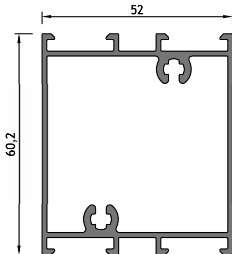
AM - 218 Travesaño
