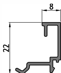
AM - 238 Contravidrio recto 8 mm Peso: 0,180 kg/m Largo: 6150 mm Paquete x 10 tiras
