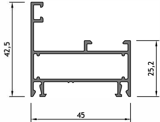
AM - 216 Marco recto Peso: 0,726 kg/m Largo: 6150 mm Paquete x 4 tiras
