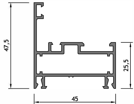
AM - 210 Marco ventana Peso: 0,786 kg/m Largo: 6150 mm Paquete x 4 tiras
