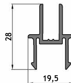
AM-246 Encuentro central de 4 hojas ventana y puerta corrediza Peso: 0,285 kg/m Largo: 6150 mm Paquete x 10 tiras
