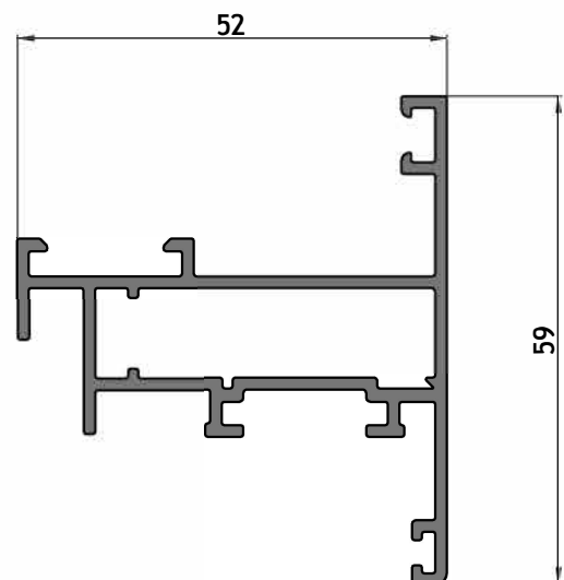
AM - 227 Hoja de ventiluz recta Peso: 0,864 kg/m Largo: 6150 mm Paquete x 3 tiras
