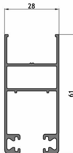
AM - 909 Hoja vidrio DVH 45° Peso: 0,794 kg/m Largo: 6150 mm Paquete x 6 tiras
