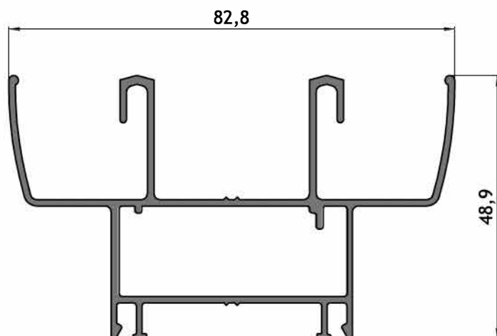
AM - 906 Marco perimetral corrediza 45° Peso: 1,183 kg/m Largo: 6150 mm Paquete x 2 tiras
