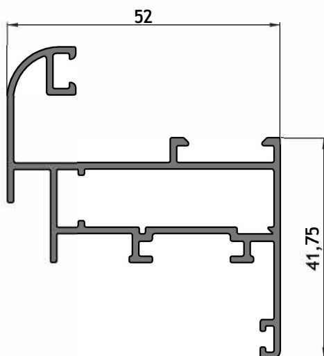
AM - 235 Hoja curva ventana de abrir doble contacto / banderola Peso: 0,902 kg/m Largo: 6150 mm Paquete x 2 tiras
