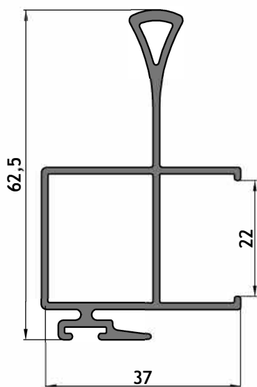
AM - 251 Parante central con tirador DVH Peso: 0,780 kg/m Largo: 6150 mm Paquete x 4 tiras
