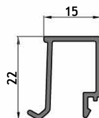
AM - 226 Contravidrio recto 15 mm Peso: 0,211 kg/m Largo: 6150 mm Paquete x 10 tiras
