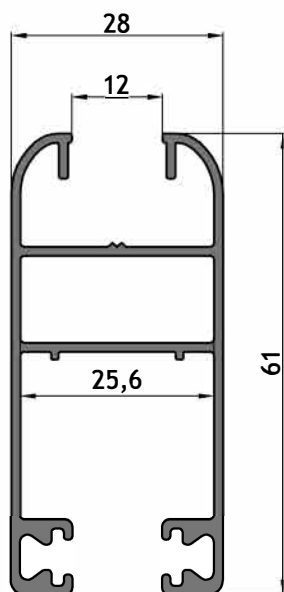
AM - 908 Hoja vidrio simple 45° Peso: 0,821 kg/m Largo: 6150 mm Paquete x 6 tiras
