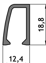
AM - 228 Tope de mosquitero Peso: 0,186 kg/m Largo: 6150 Paquete x 10 tiras
