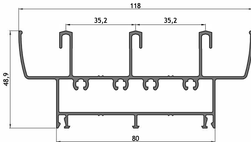
AM - 240 Umbral y dintel 3 guías Peso: 1,652 kg/m Largo: 6150 mm Paquete x 2 tiras
