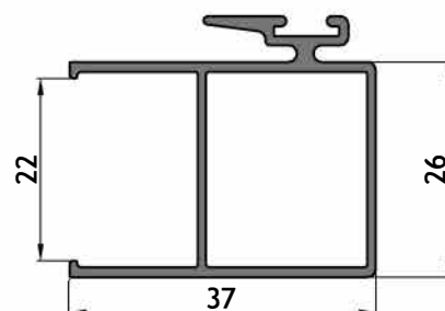
AM - 250 Parante central DVH Peso: 0,567 kg/m Largo: 6150 mm Paquete x 6 tiras
