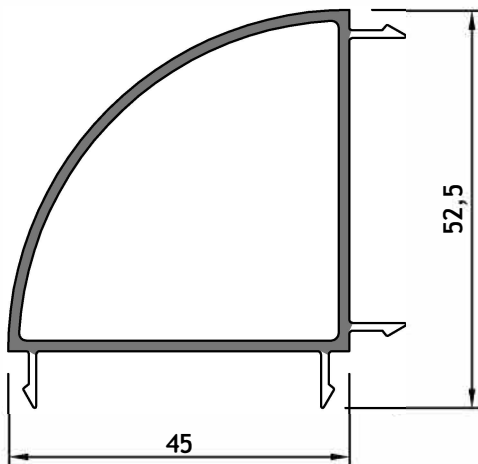
AM - 262 Acople a 90° Peso: 0,675 kg/m Largo: 6150 mm Paquete x 2 tiras
