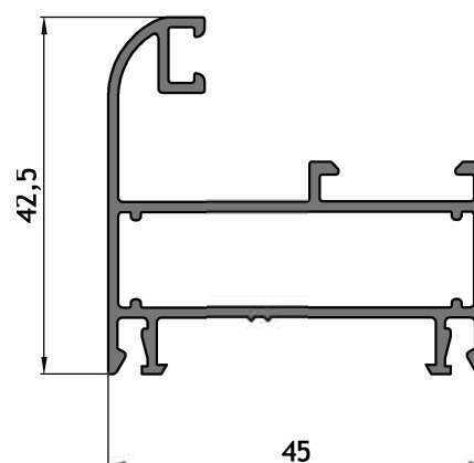
AM - 229 Marco curvo Peso: 0,764 kg/m Largo: 6150 mm Paquete x 4 tiras
