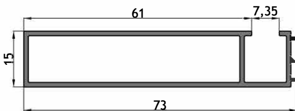
AM - 901 Premarco 73 Peso: 0,575 kg/m Largo: 6150 mm Paquete x 10 tiras
