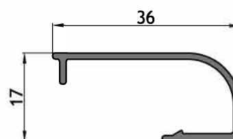
AM - 257 Contravidrio curvo 36 mm Peso: 0,235 kg/m Largo: 6150 mm Paquete x 10 tiras
