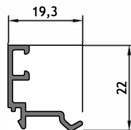
AM - 220 Contravidrio exterior puerta rebatir Peso: 0,176 kg/m Largo: 6150 mm Paquete x 10 tiras
