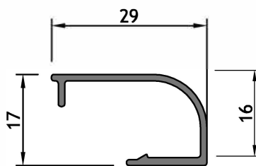
AM - 230 Contravidrio curvo 29 mm Peso: 0,213 kg/m Largo: 6150 mm Paquete x 10 tiras
