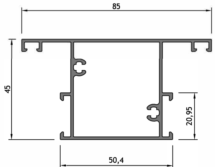
AM - 615 Travesaño de puerta de 45 mm Peso: 0,980 kg/m Largo: 6150 mm Paquete x 2 tiras
