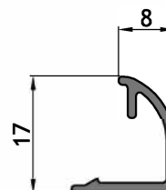
AM - 233 Contravidrio curvo 8 mm Peso: 0,135 kg/m Largo: 6150 mm Paquete x 10 tiras
