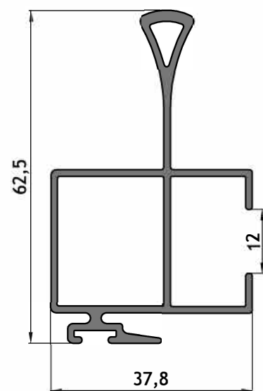
AM - 208 Parante central con tirador Peso: 0,802 kg/m Largo: 6150 mm Paquete x 4 tiras
