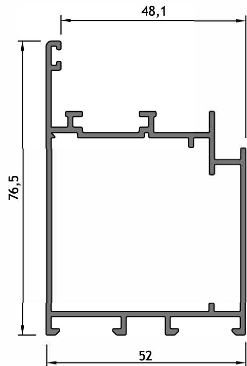
AM - 214 Parante
