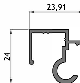
AM - 254 Tapacintas hembra Peso: 0,295 kg/ml Largo: 6150 mm Paquete x 10 tiras
