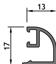
AM - 237 Contravidrio curvo puerta rebatir Peso: 0,181 kg/m Largo: 6150 mm Paquete x 10 tiras
