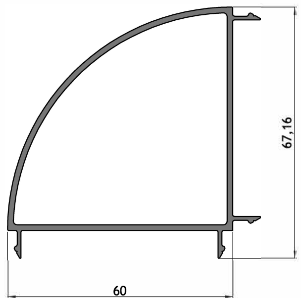
AT-069 Acople a 90° Peso: 0,927 kg/m
