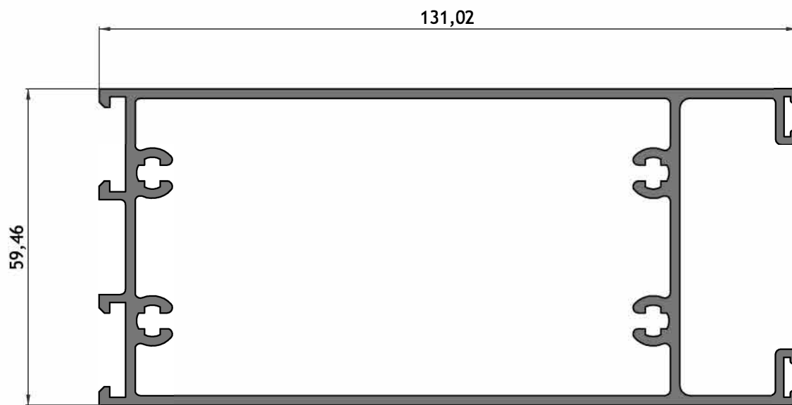
AT-043 Zócalo de puerta Peso: 2,319 kg/m
