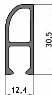
AT-039 Tope de mosquitero Peso: 0,330 kg/m
