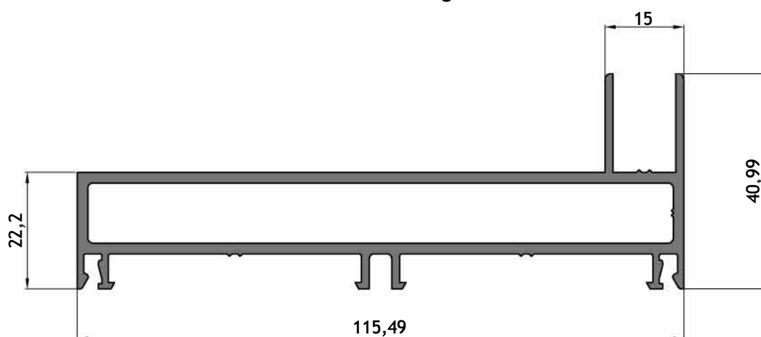
AT-081 Umbral de 3 guías Peso: 2,908 kg/m
