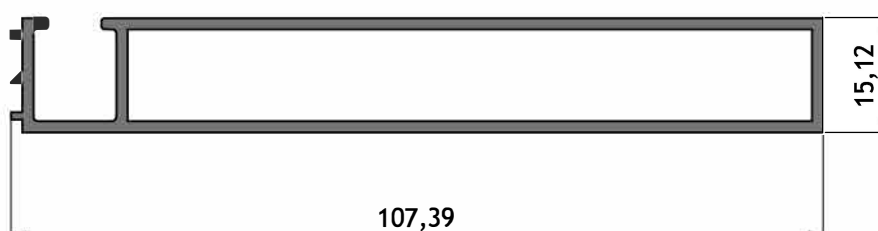
AT-079 Premarco corrediza de 3 hojas Peso: 0,982 kg/m
