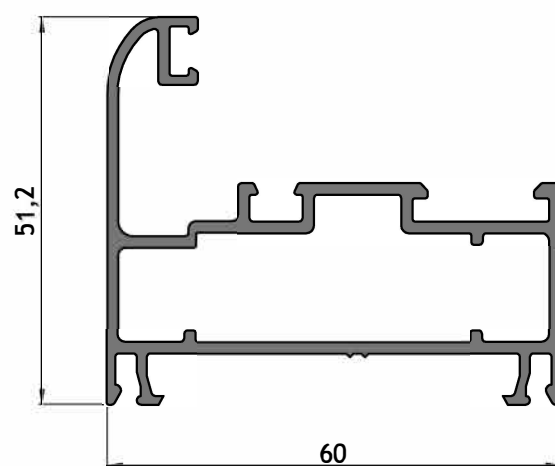
AT-055 Marco curvo paño fijo y ventana de abrir Peso: 1,022 kg/m
