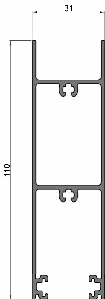
AT-074 Zócalo alto puerta corrediza DVH Peso: 1,370 kg/m
