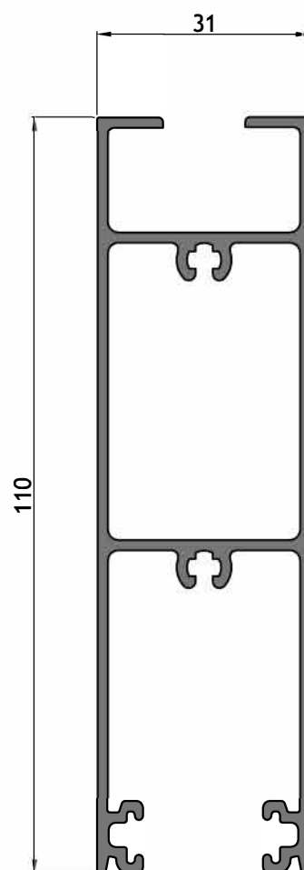
AT-062 Zócalo alto puerta corrediza Peso: 1,470 kg/m
