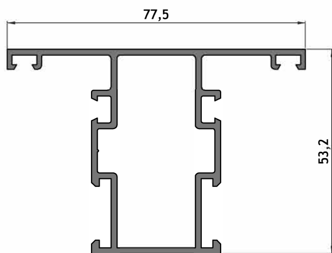
AT-060 Travesaño de paño fijo Peso: 1,091 kg/m
