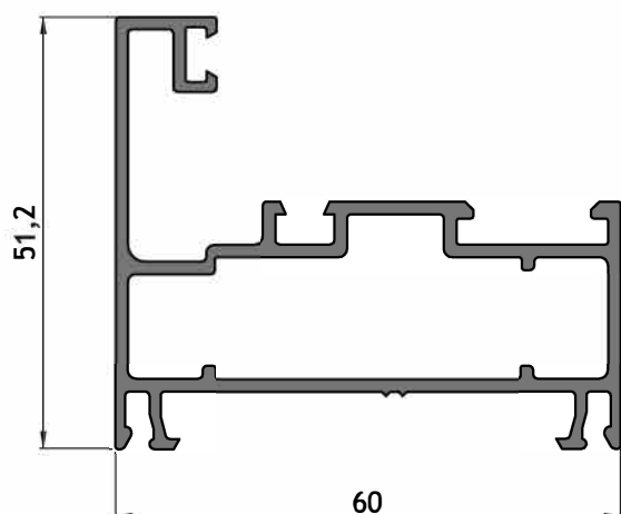
AT-059 Marco recto paño fijo y ventana de abrir Peso: 1,040 kg/m
