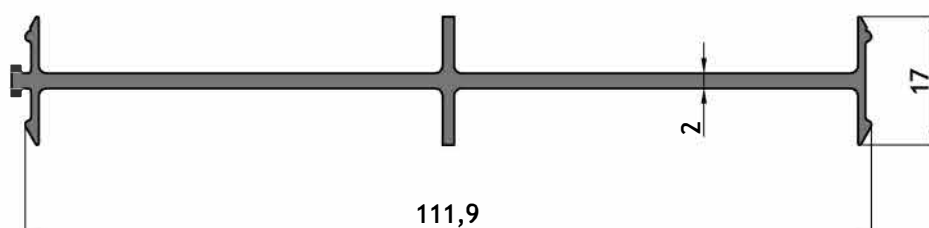
AT-080 Jamba de marco Peso: 1,702 kg/m
