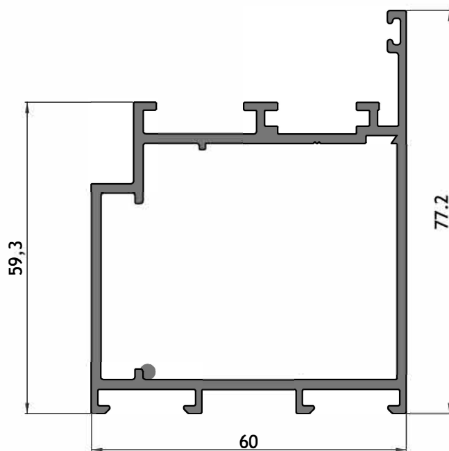
AT-041 Hoja puerta de rebatir Peso: 1,380 kg/m
