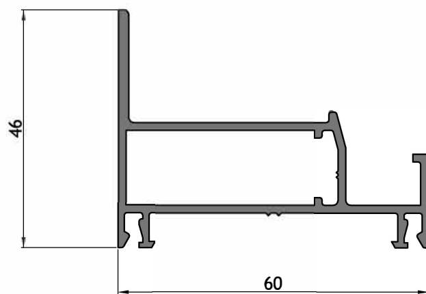
AT-057 Marco proyectante Peso: 0,836 kg/m
