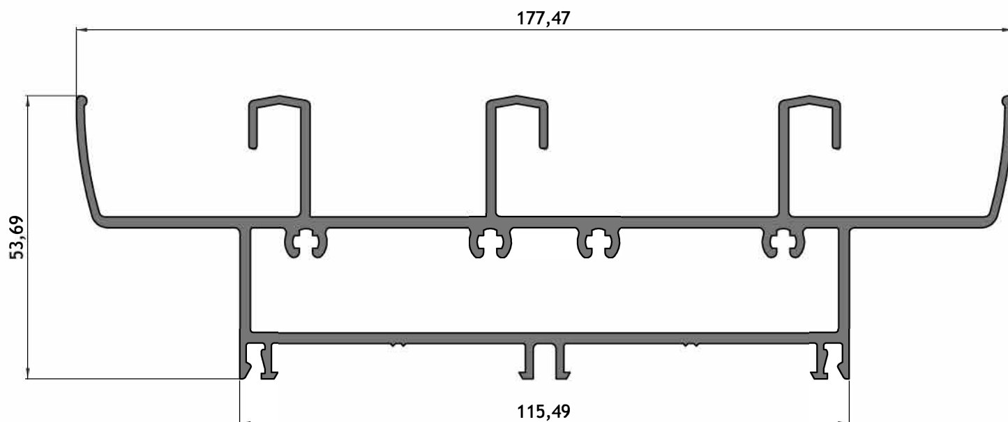
AT-081 Umbral de 3 guías Peso: 2,908 kg/m
