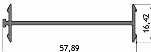
AT-067 Perfil de acople Peso: 0,324 kg/m
