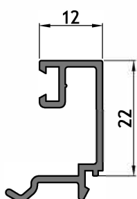
AT-049 Contravidrio exterior Peso: 0,230 kg/m
