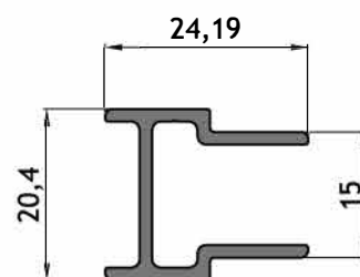
AT-965 Encuentro central corrediza 4 hojas Peso: 0,290 kg/m
